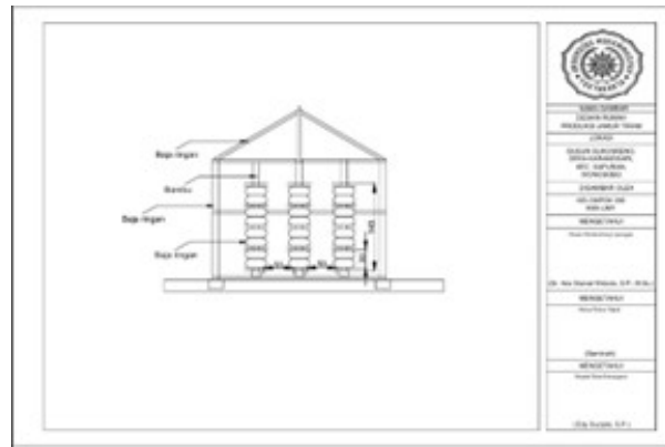
Gambar 6. Desain rumah produksi jamur tiram
